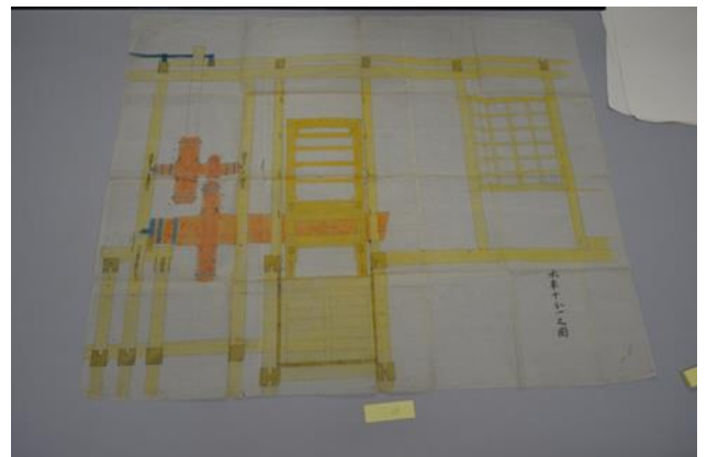
写真4 水車十分之一図
